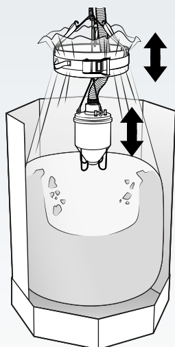
Tête d'aspiration oscillante et tension de sac
